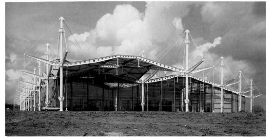
Norman Foster: Renault Központ, Swindon, Anglia, 1983.
