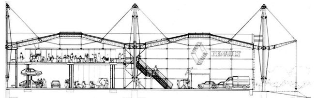
Norman Foster: Renault Központ, Swindon, Anglia, 1983.
