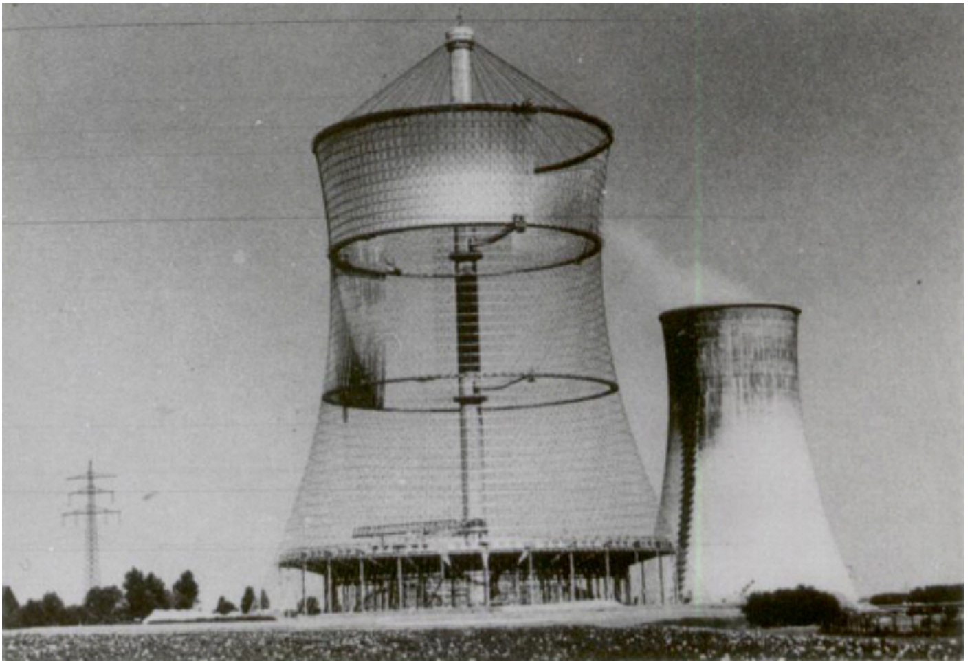
Hűtőtorony a külső héjazat szerelése közben
