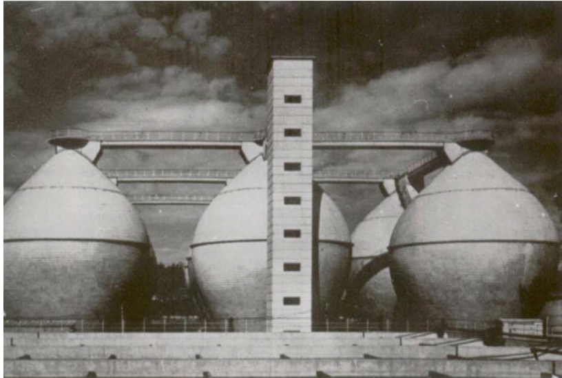
Ülepítők Németország, Düsseldorf-Süd, Kanal und Wasserbaumat, Düsseldorf, 1969
