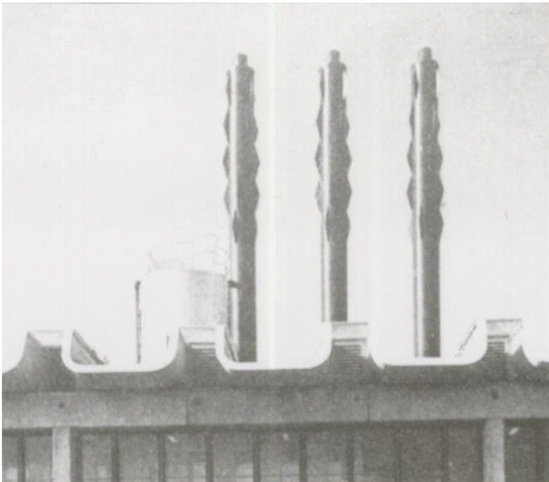
Örvényleválasztást szabályozó hármasspirál
